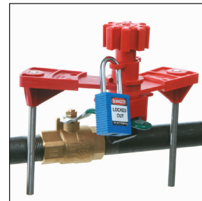
Use dos brazos de bloqueo para bloquear válvulas de 3, 4 o 5 vías, o para bloquear válvulas en la posición de encendido, apagado.
