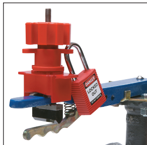
Se coloca en manijas de mariposa, evitando que el gatillo de la manija sea presionado.
